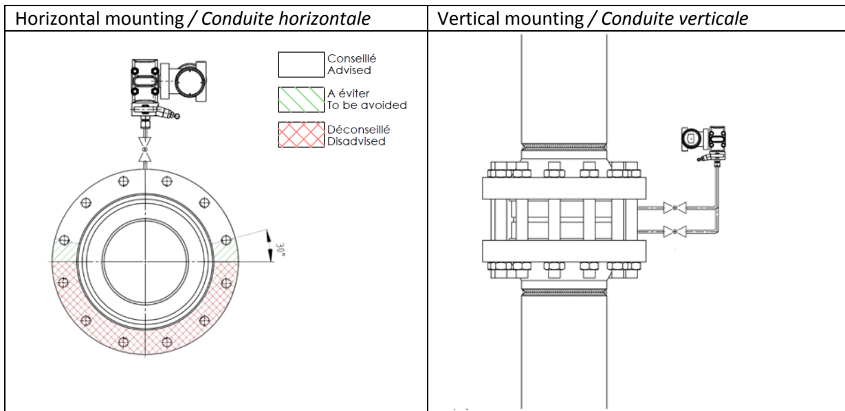
Fig 6 : Transmitter mounting for gas applications Fig 6 : Montage du transmetteur pour une application avec un fluide gazeux
