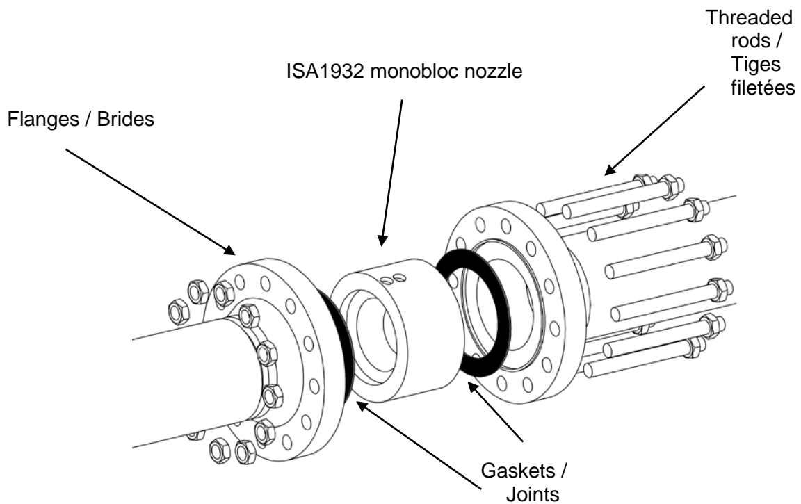
Fig 4 : Assembly of an ISA1932 monobloc nozzle between flanges Fig 4 : Montage d'une tuyère ISA1932 monobloc entre brides
