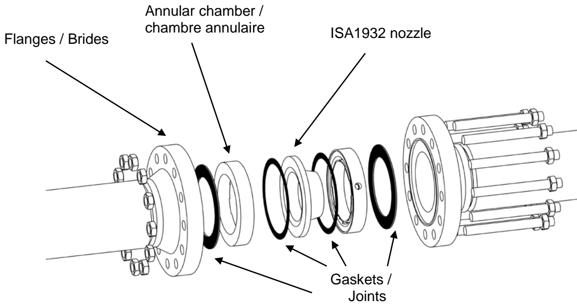
Fig 3 : Assembly of an ISA1932 nozzle in annular chamber elements and between flanges Fig 3 : Montage d'une tuyère ISA1932 entre éléments de chambre annulaire et entre brides
